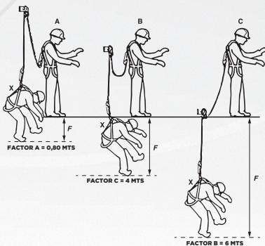
Para sujeción de posicionamiento.
